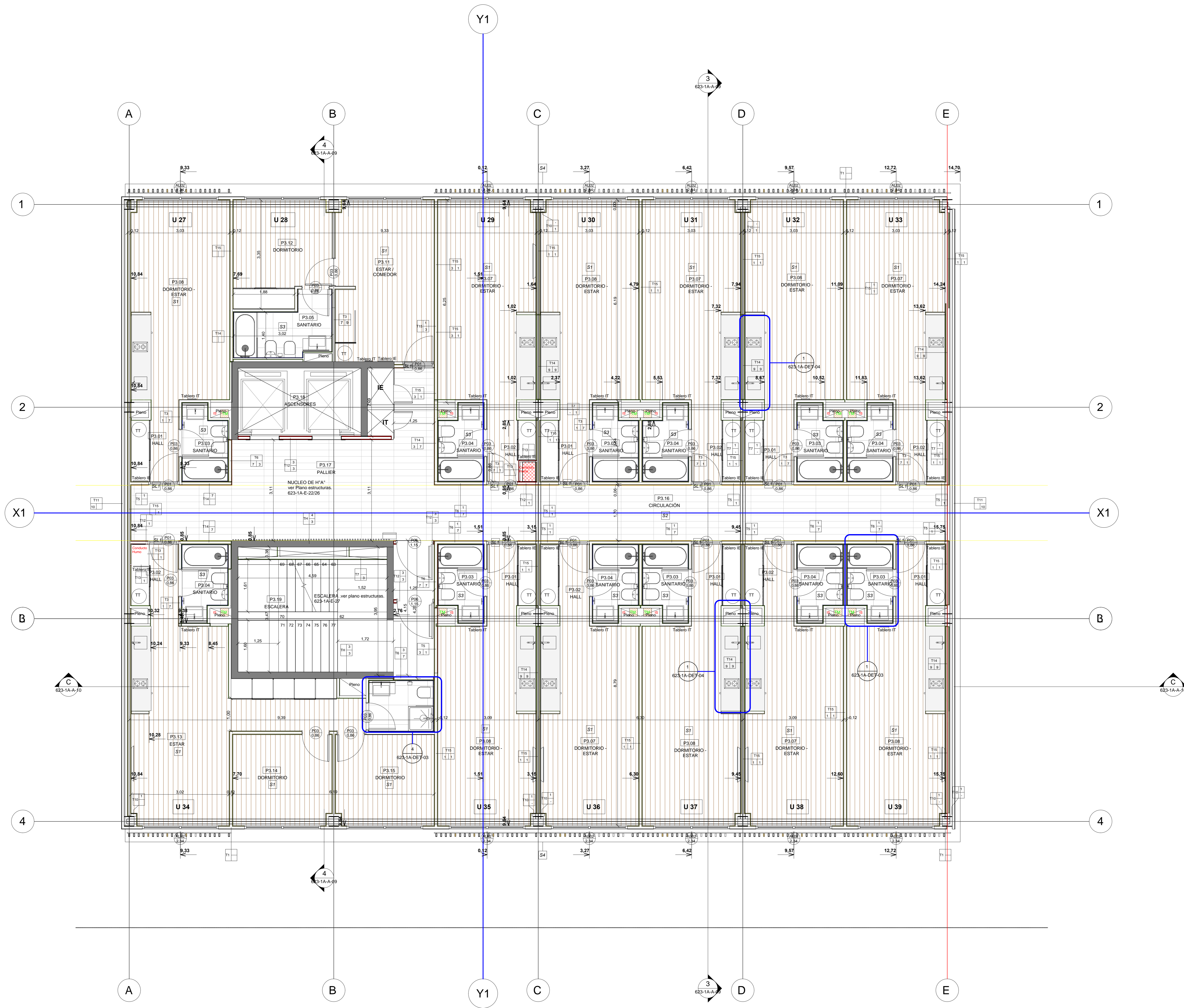
1 03-REPLANTEO TERCER PISO Esc. 1:50
