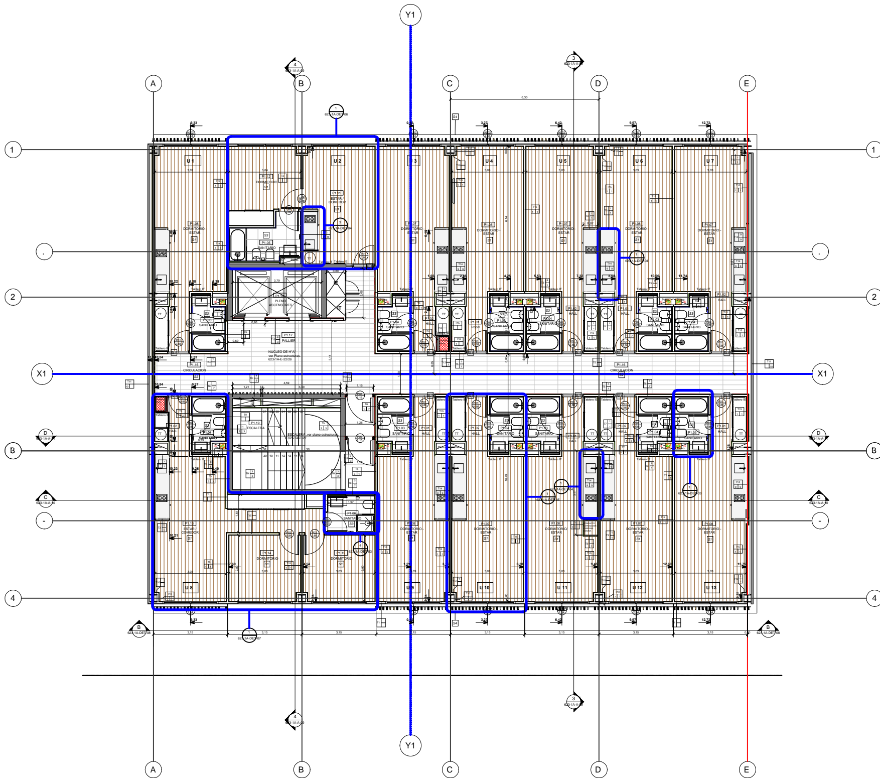
1 01-REPLANTEO PRIMER PISO Escala: 1:50
